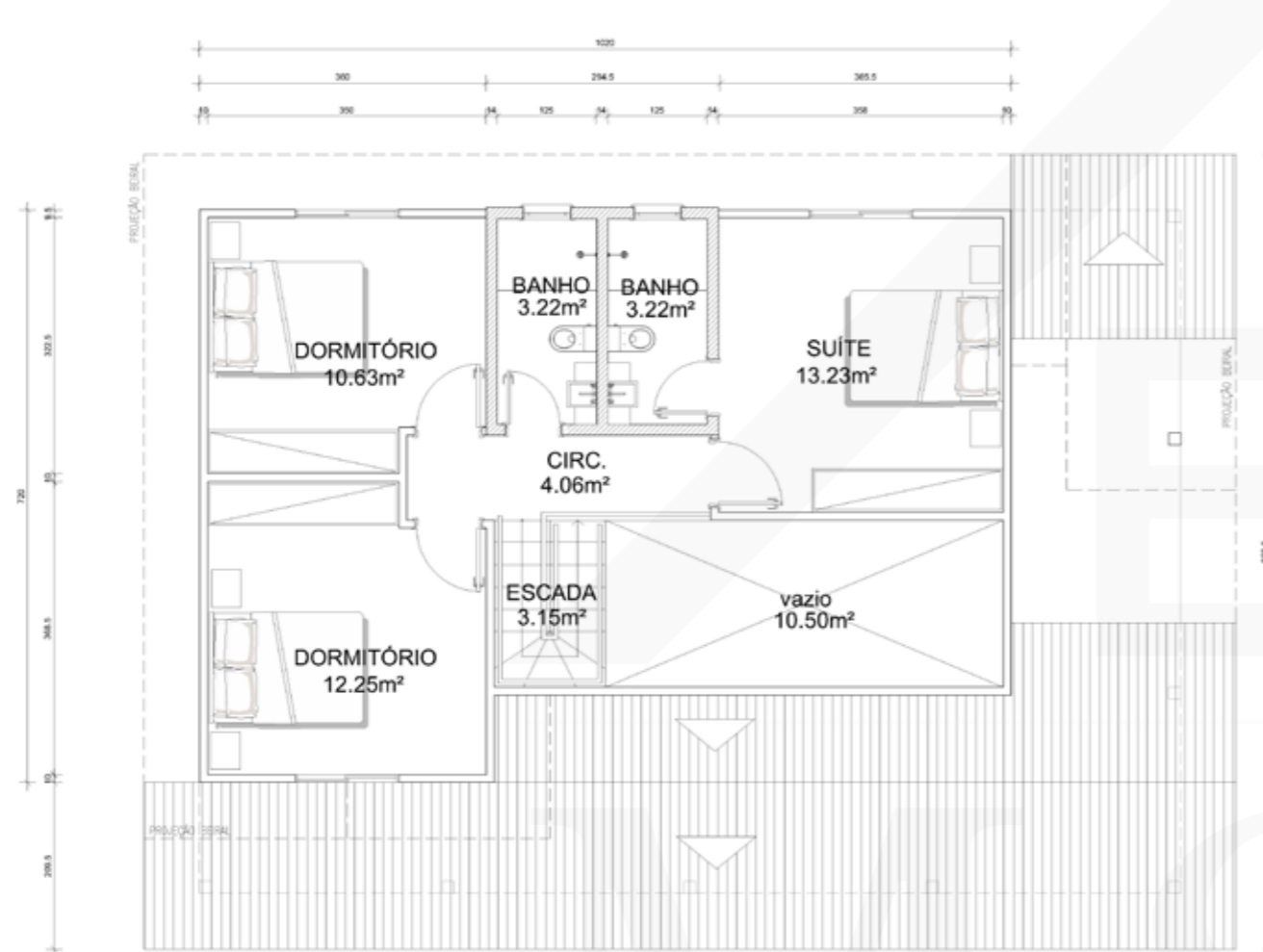
PLANTA PAV. SUPERIOR ÁREA=55.76m 2
