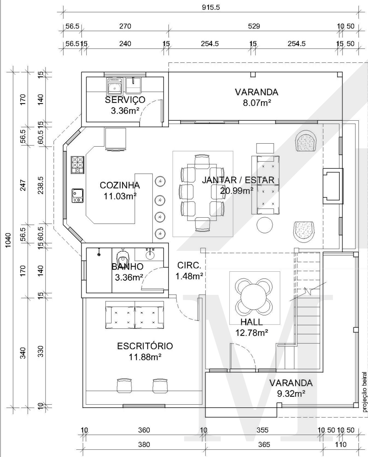
PLANTA BAIXA PAV. TÉRREO ÁREA= 88.10m²
