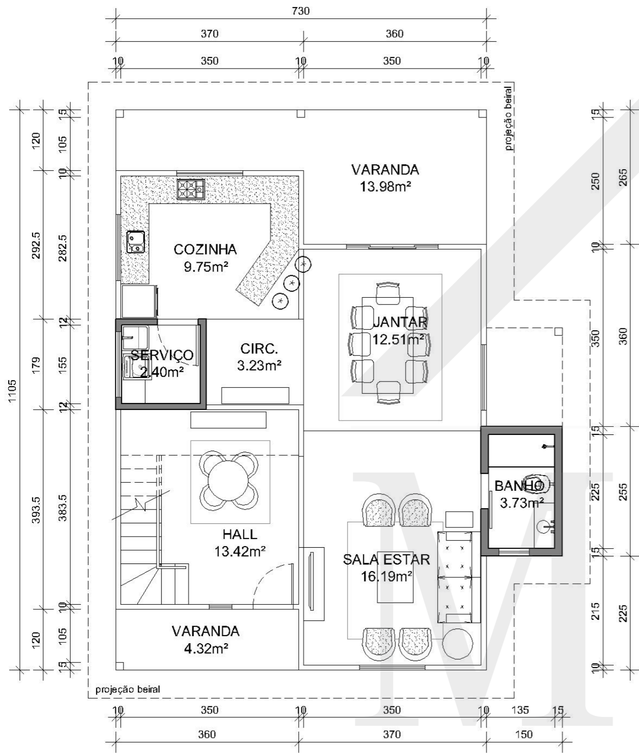
PLANTA BAIXA PAV. TÉRREO ÁREA= 84.50m 2
