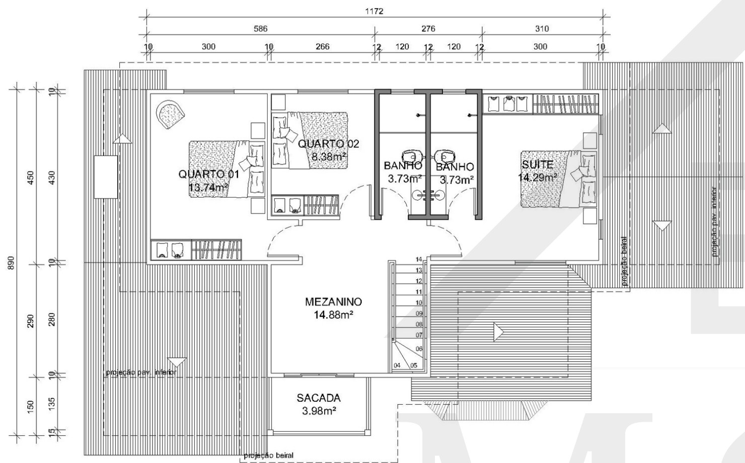
PLANTA BAIXA PAV. SUPERIOR
