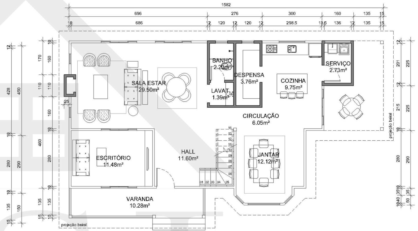
PLANTA BAIXA PAV. TÉRREO
