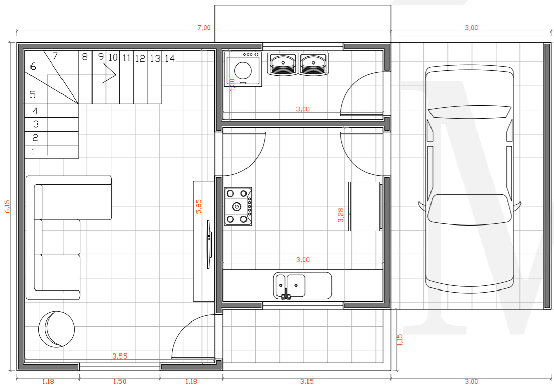
Pav Inferior esc: 1/50 área: 54,10m 2
